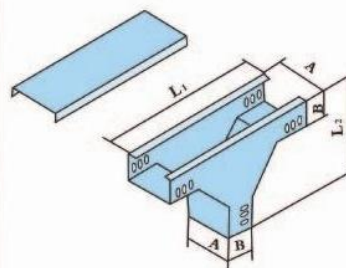
XQJ-C-03B 型上垂直三通
