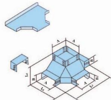
XQJ-C-04B 型上垂直四通
