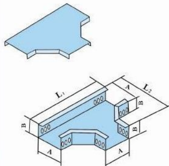
XQJ-C-03A 型水平三通
