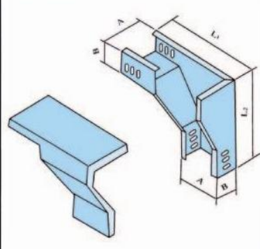
XQJ-C-05E 型垂直右上弯通
