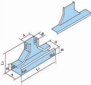
XQJ-C-03E 型下侧垂直三通
