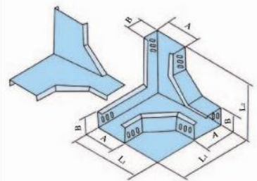
XQJ-C-03G 型下角垂直三通
