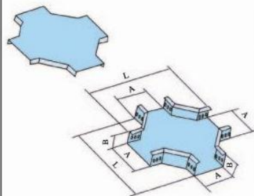
XQJ-C-04A 型水平四通
