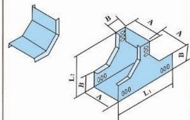
XQJ-C-03C 型下垂直三通
