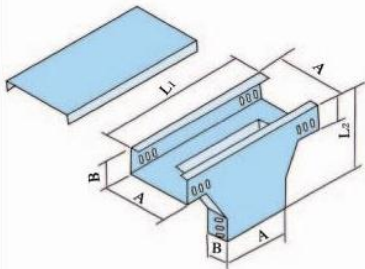
XQJ-C-03D 型上侧垂直三通
