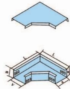
XQJ-C-02A 型水平弯通
