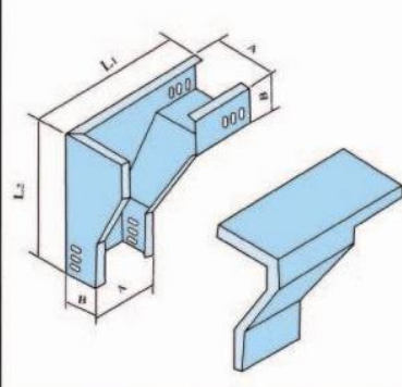
XQJ-C-05C 型垂直左上弯通
