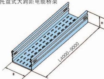
托盘式大跨距电缆桥架
