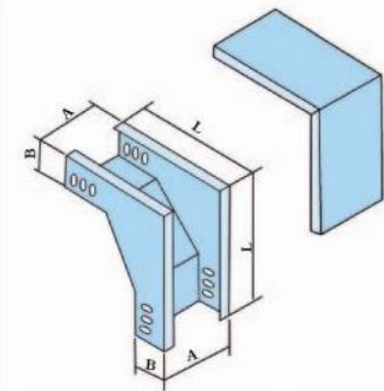
XQJ-C-05A 型垂直上弯通
