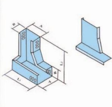
XQJ-C-05D 型垂直左下弯通
